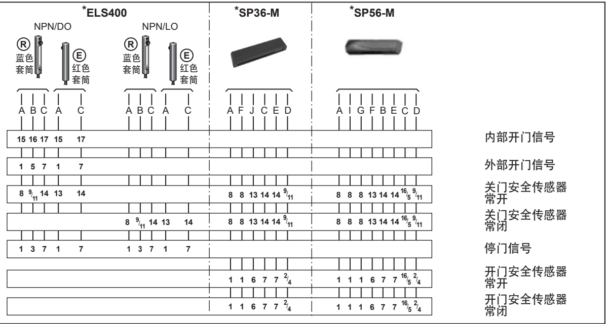
控制单元端口接线
