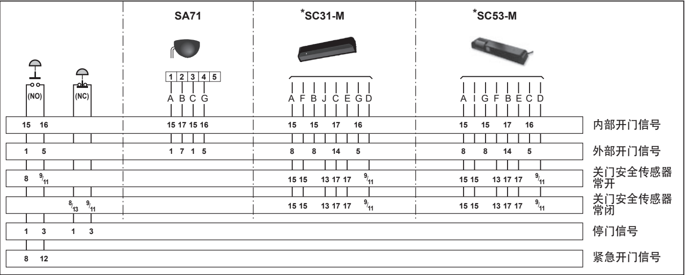
控制单元端口接线
